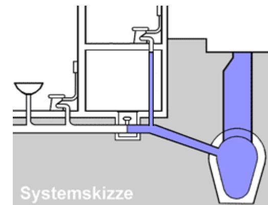
Rückstauverschluss
