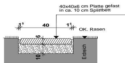
Einbau Schnitt
