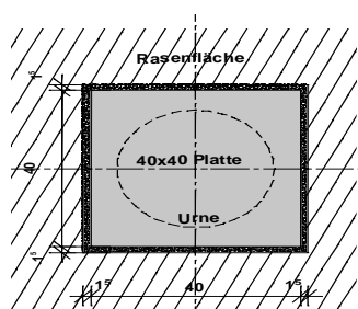
Einbau Aufsicht
